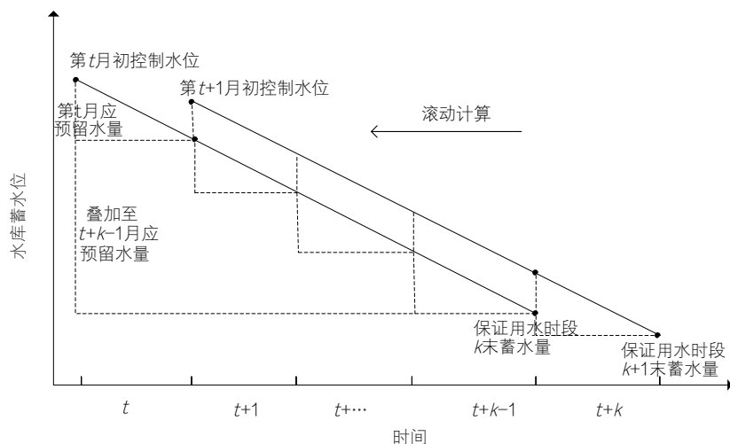
图3 供水调度分级控制计算示意
